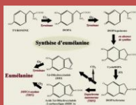
Synthèse de l'eumélanine
