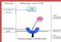
Mécanisme de la synthèse de l'eumélanine d'après S. Danvy & al. 08/2011
